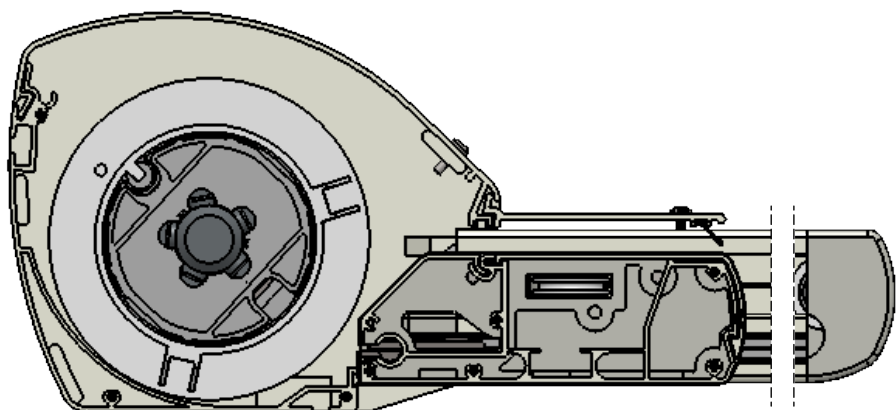
Doorsnede
